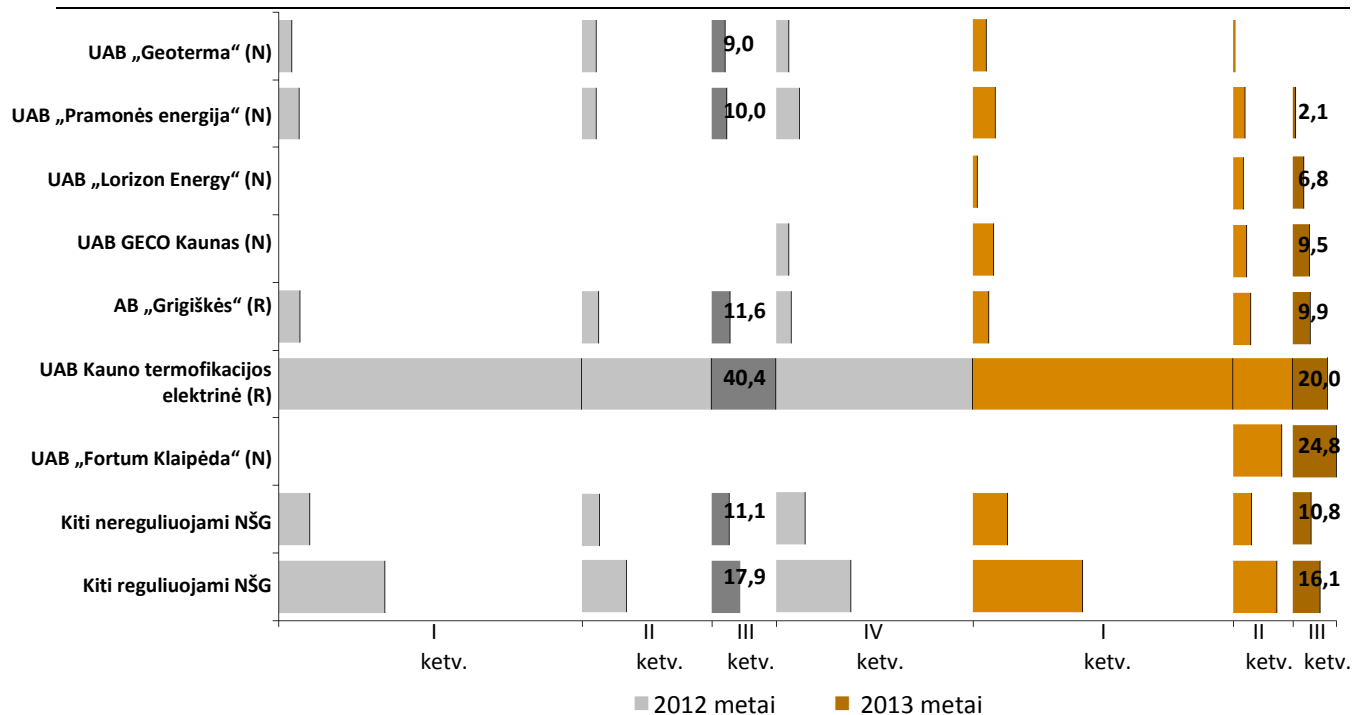
1 pav. Didžiausių nepriklausomų šilumos gamintojų pagamintos šilumos rinkos dalys (proc.), 2012 I ketv. – 2013 m. III ketv.
