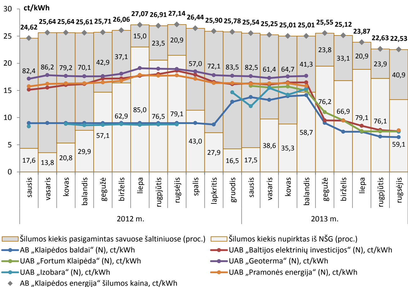
13 pav. Nepriklausomų šilumos gamintojų parduotos šilumos dalis AB „Klaipėdos energija“ patiektos šilumos struktūroje, proc., parduotos šilumos kaina ir AB „Klaipėdos energija“ parduodamos šilumos kaina, ct/kWh, be PVM, 2012 m. sausis – 2013 m. rugsėjis.
