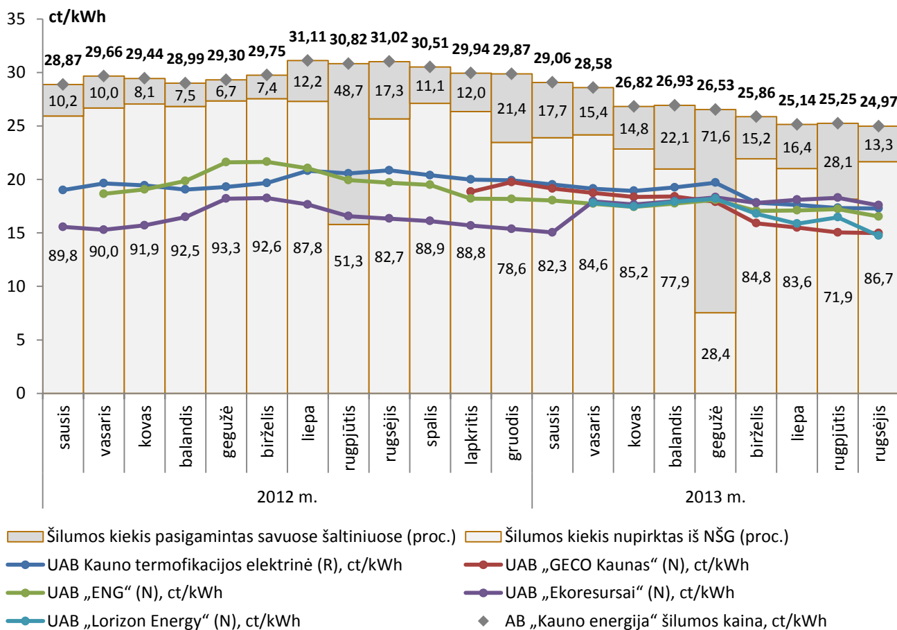
12 pav. Nepriklausomų šilumos gamintojų parduotos šilumos dalis AB „Kauno energija“ patiekto šilumos struktūroje, proc., parduotos šilumos kaina ir AB „Kauno energija“ parduodamos šilumos kaina, ct/kWh, be PVM, 2012 m. sausis – 2013 m. rugsėjis.
