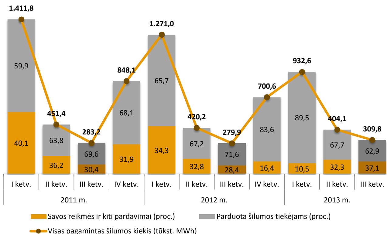
6 pav. Nepriklausomų šilumos gamintojų pagamintos šilumos struktūra pagal panaudojimą, 2011 m. I ketv. – 2013 m. III ketv.
