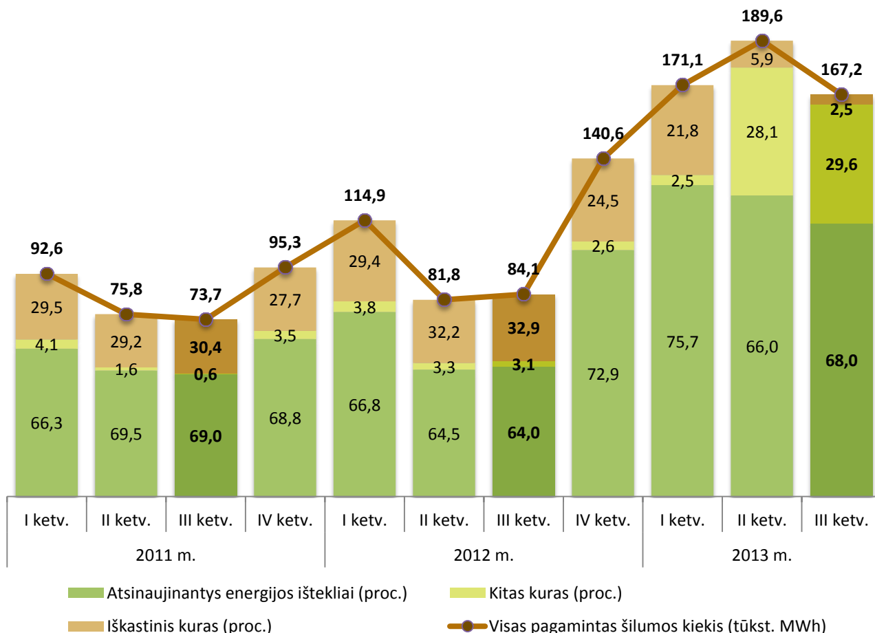
5 pav. Nereguliuojamų nepriklausomų šilumos gamintojų pagamintos šilumos kiekis pagal kuro rūšis (proc.) ir bendras pagamintas kiekis (tūkst. MWh), 2011 m. I ketv. – 2013 m. III ketv.
