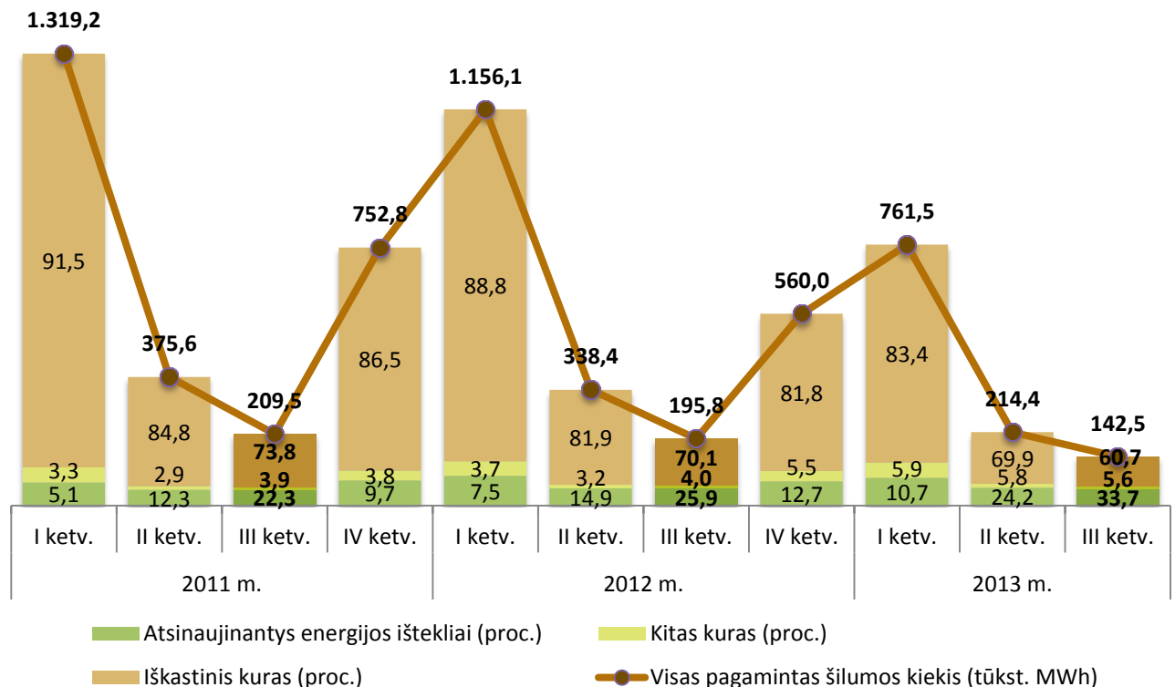
4 pav. Reguluojamų nepriklausomų šilumos gamintojų pagamintos šilumos kiekis pagal kuro rūšis (proc.) ir bendras pagamintas kiekis (tūkst. MWh), 2011 m. I ketv. – 2013 m. III ketv.
