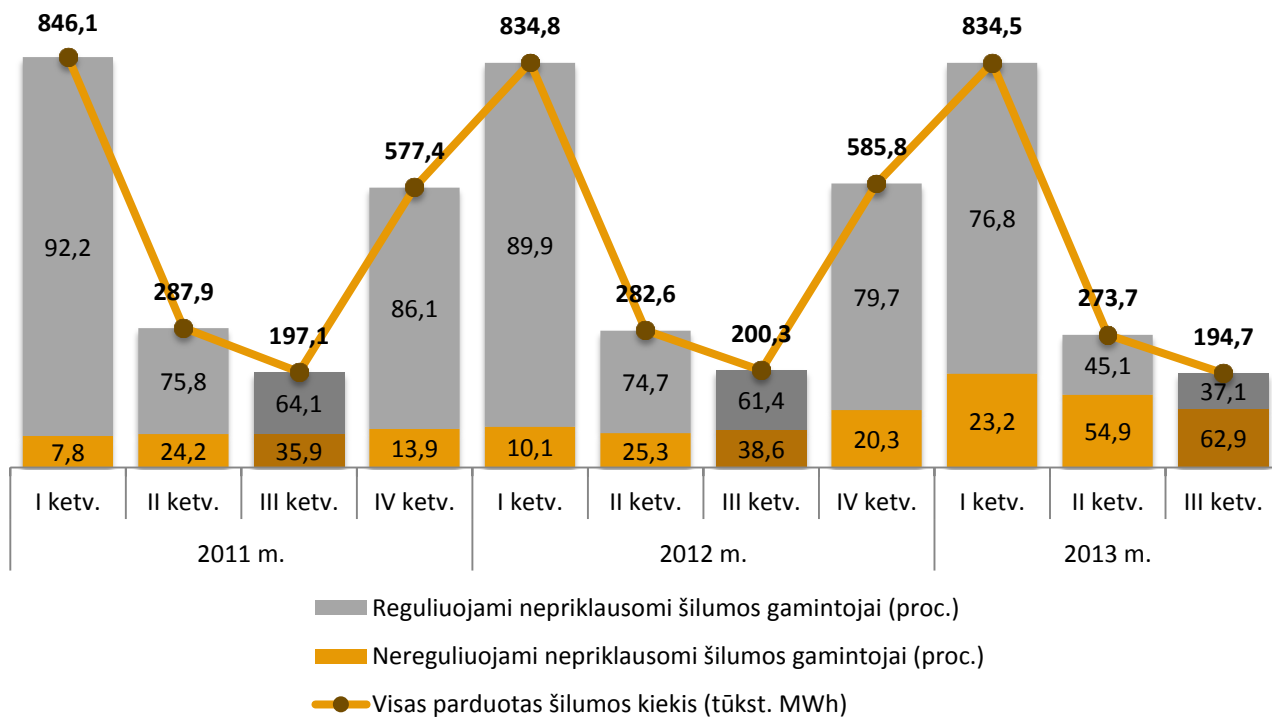
7 pav. Nepriklausomų šilumos gamintojų į Komisijos licencijuojamų šilumos tiekėjų tinklus patiektos šilumos kiekis, 2011 m. I ketv. – 2013 m. III ketv.
