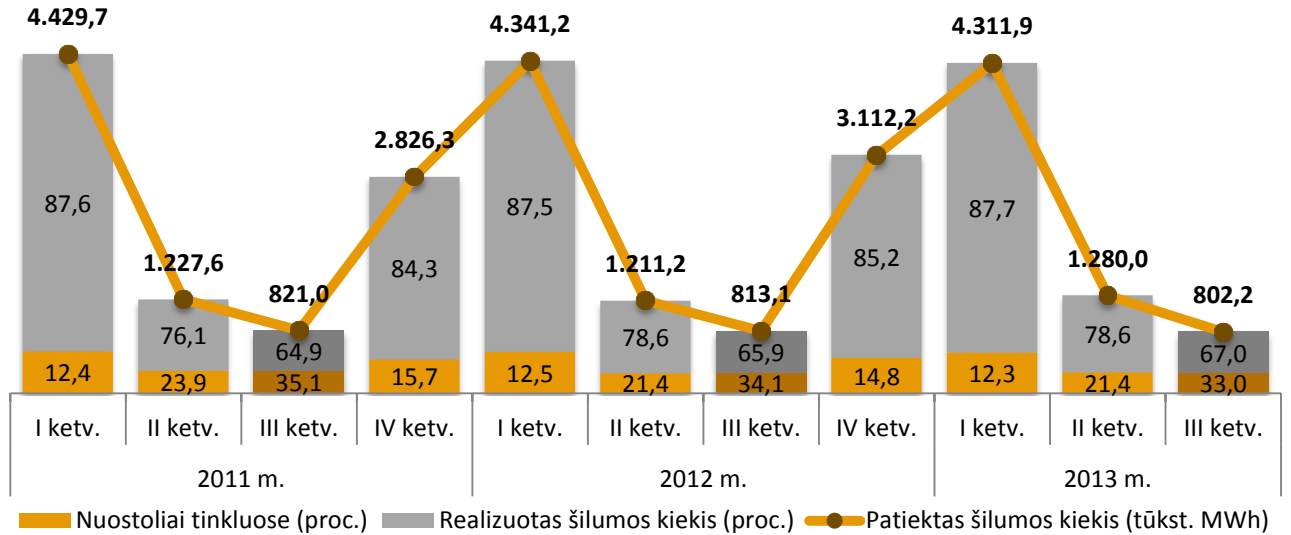
10 pav. Komisijos licencijuojamų šilumos tiekėjų vartotojams patiekto šilumos kiekio struktūra, 2011 m. I ketv. – 2013 m. III ketv.
