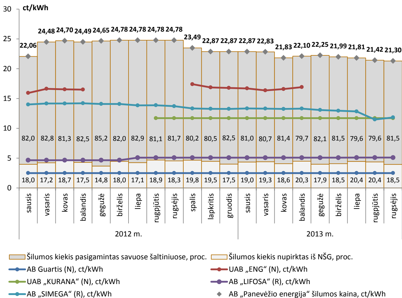
14 pav. Nepriklausomų šilumos gamintojų parduotos šilumos dalis AB „Panevėžio energija“ patiektos šilumos struktūroje, proc., parduotos šilumos kaina ir AB „Panevėžio energija“ parduodamos šilumos kaina, ct/kWh, be PVM, 2012 m. sausis – 2013 m. rugsėjis.
